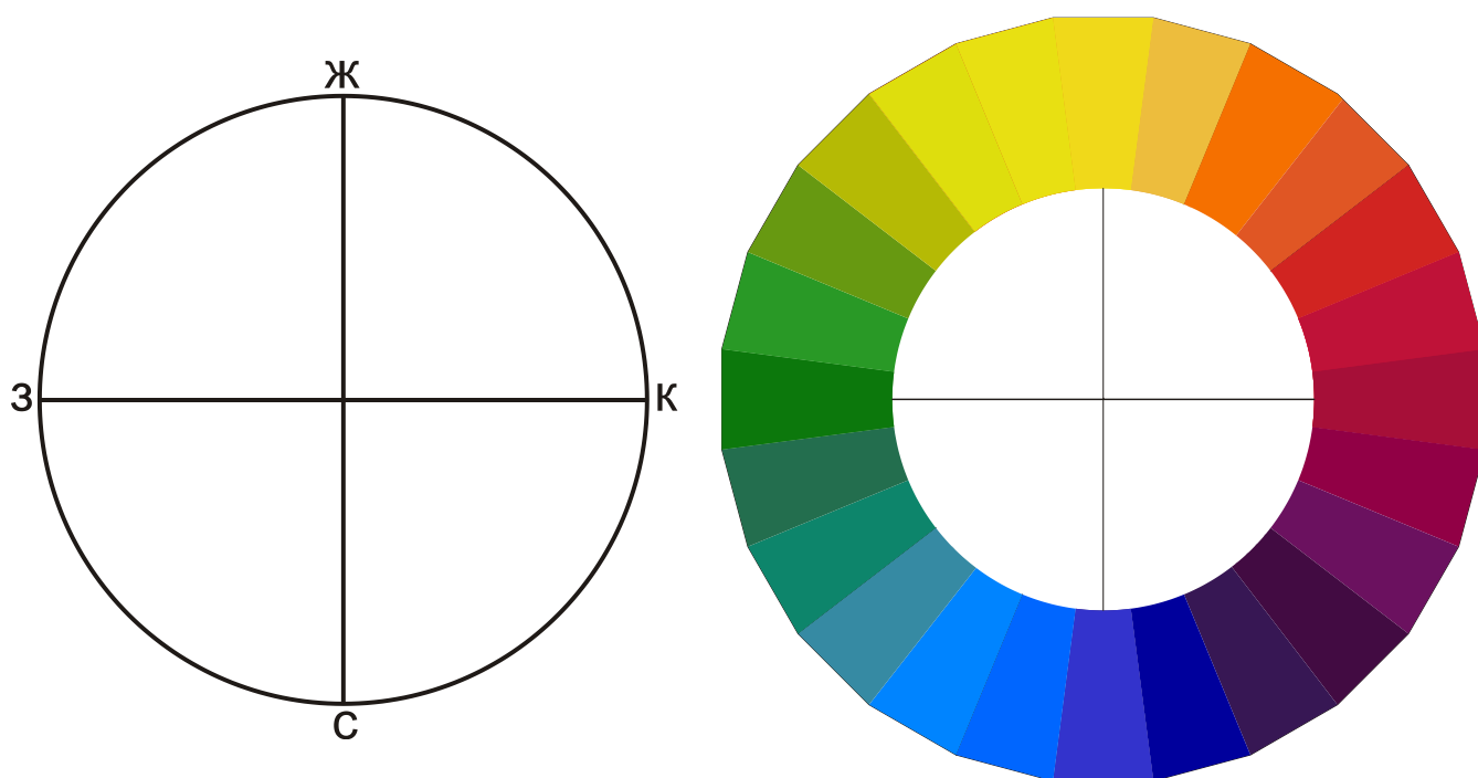
Рисунок 16 Цветовой круг
